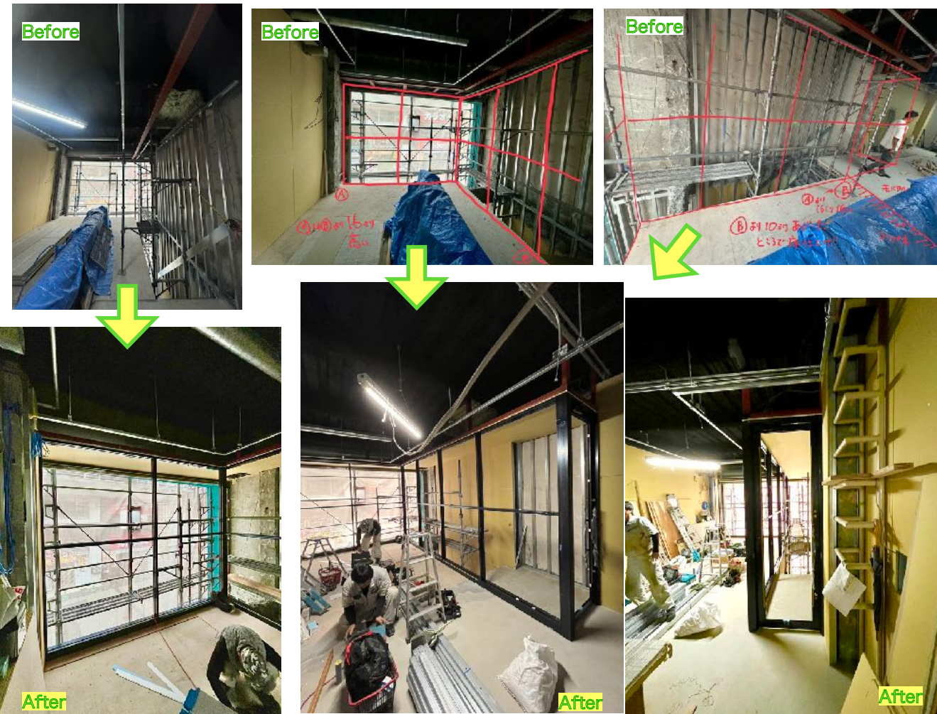
(株)小川技硝 藤井様分 姫路駅前現場 STフロント100コーナーFIX付片開丁番ドア
